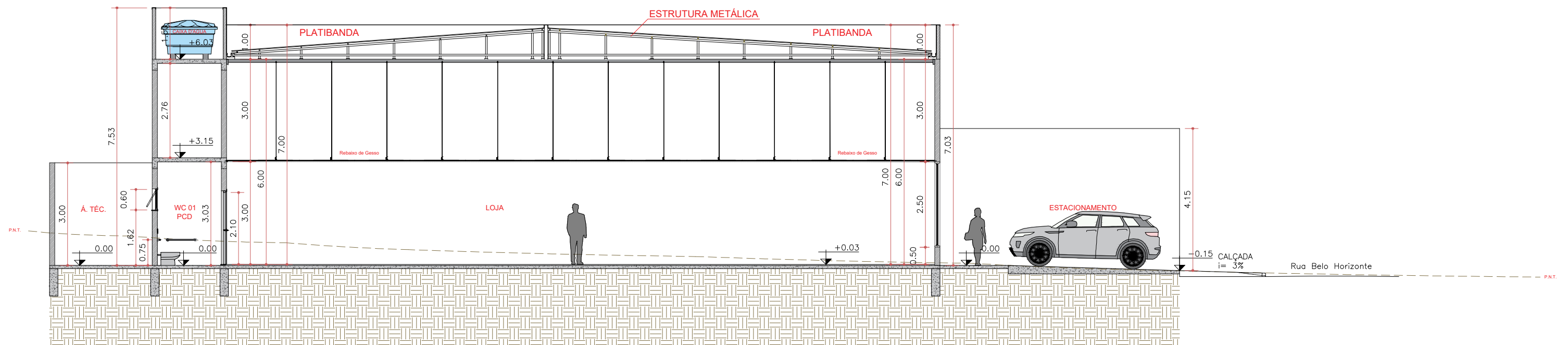
CORTE AA SEM ESCALA
